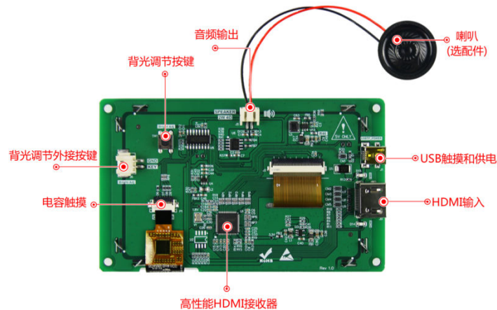
图 1-2 硬件配置图
